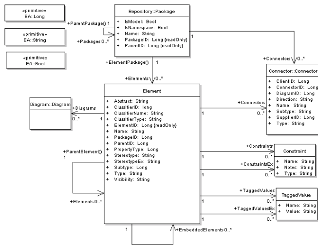
Abbildung 2: Auszug aus dem EA Metamodell
