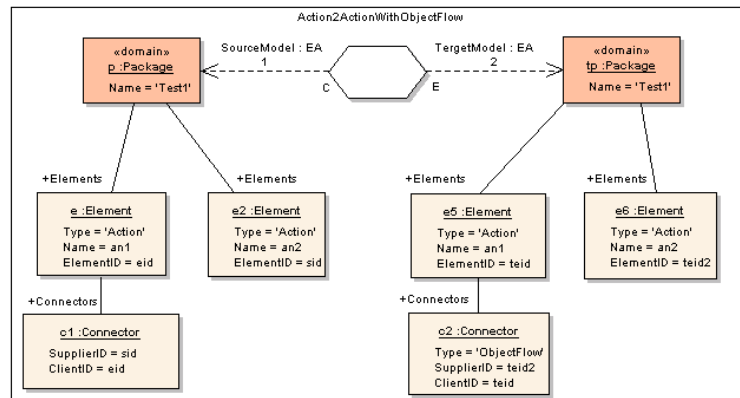
Abbildung 1: Beispiel einer mit Enterprise Architect erstellten QVT Relation
