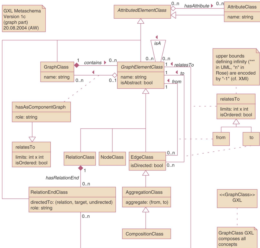
Fig. 16. GXL metaschema.
